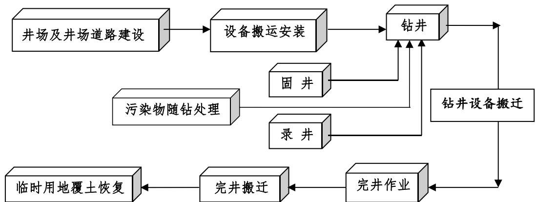
图 2-1 项目施工作业过程示意图
