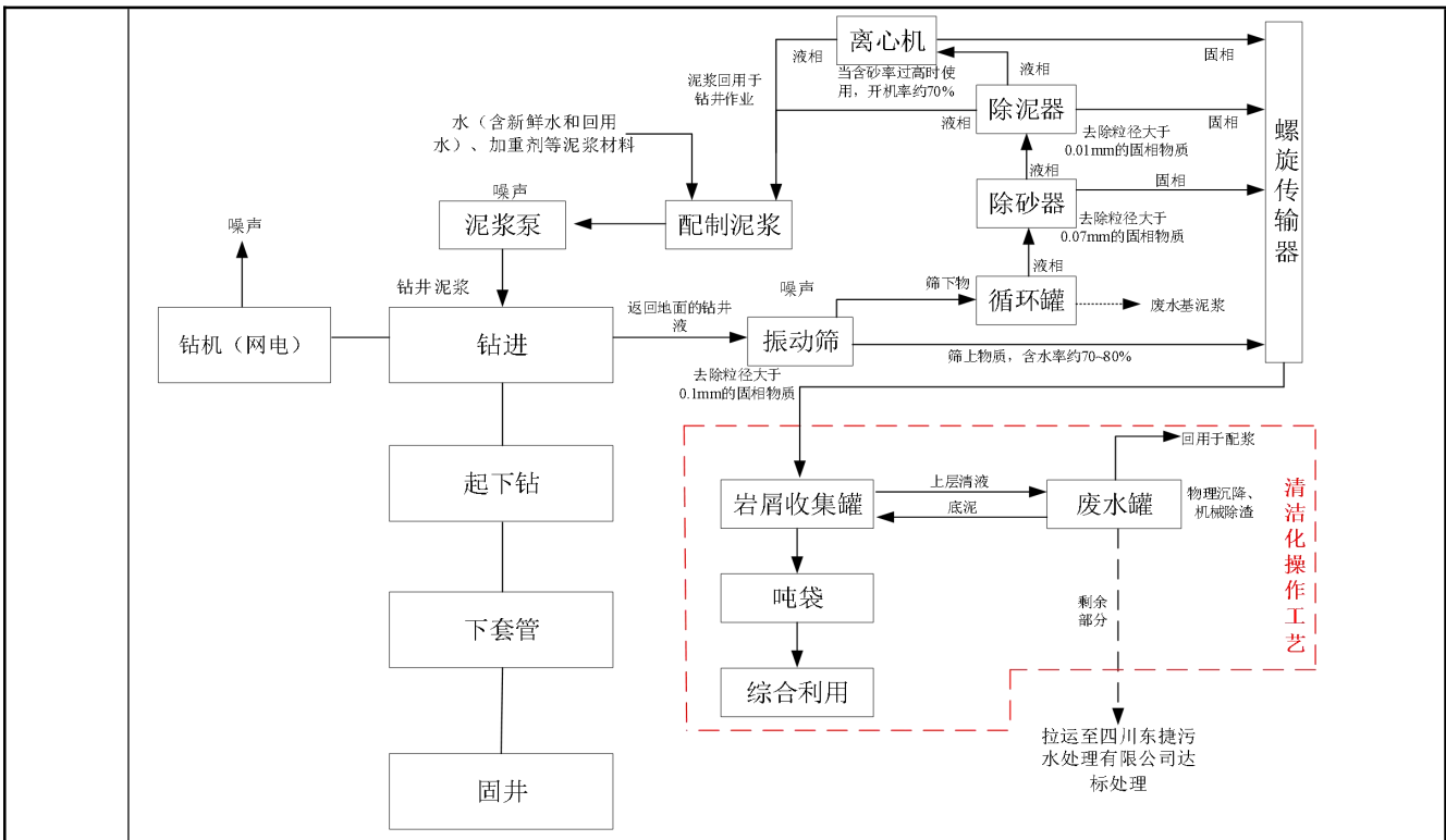
图 2-7 水基钻井液钻阶段作业流程及产污节点框图
