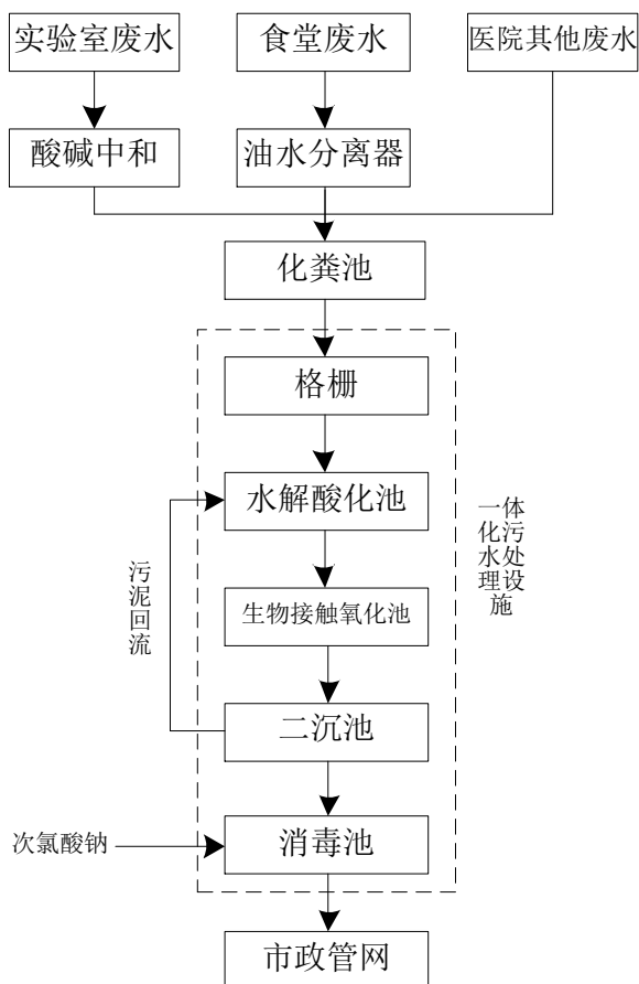
图 4-5 本项目废水处理工艺流程图
