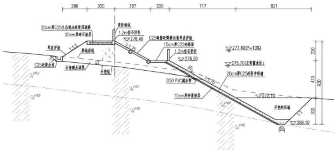
图 2-1 斜坡式堤型图
