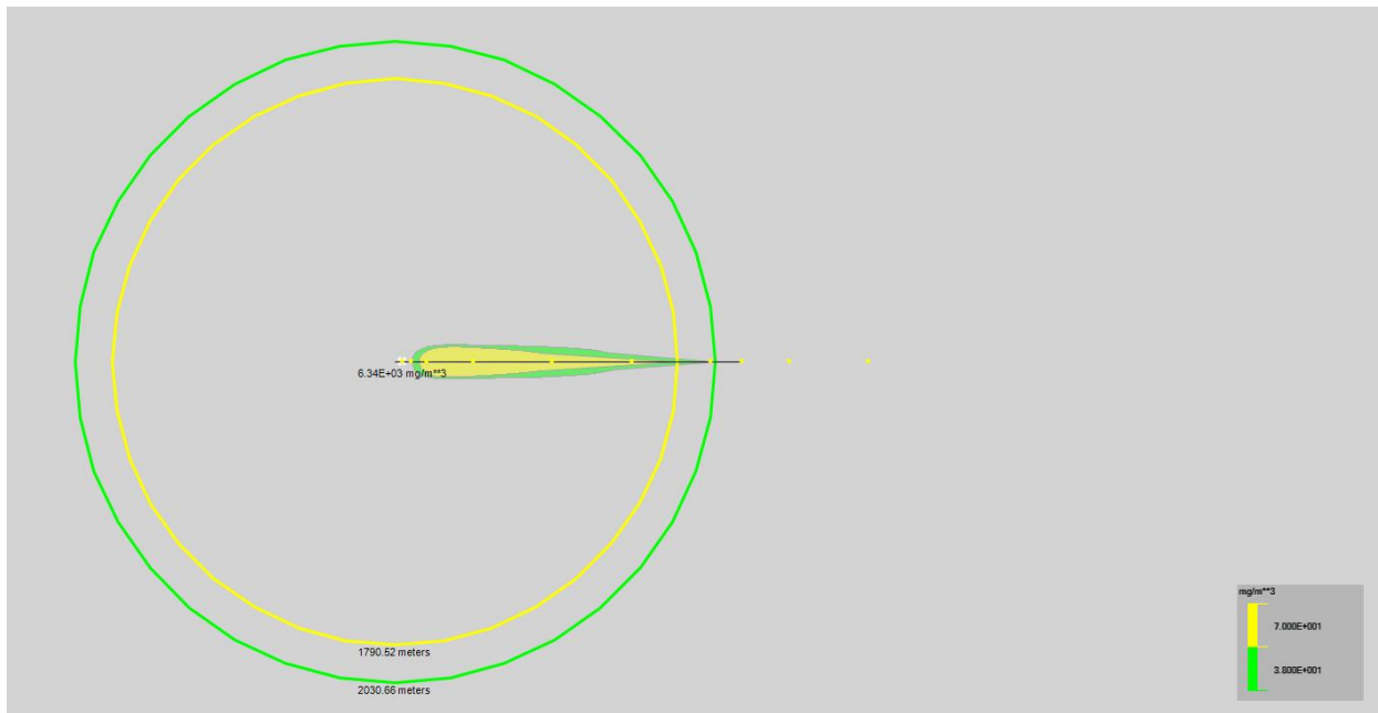
图 4-1 垂直喷射事故结果示意图（H 2 S）
