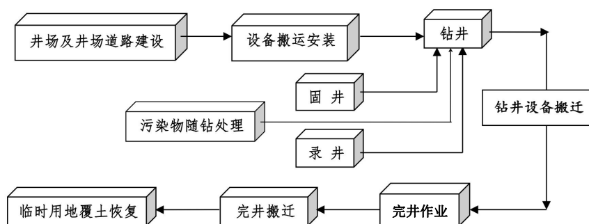
图 2-1 项目施工作业过程示意图
