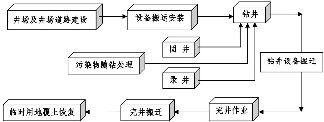
图 2-1 项目钻井施工作业过程示意图
