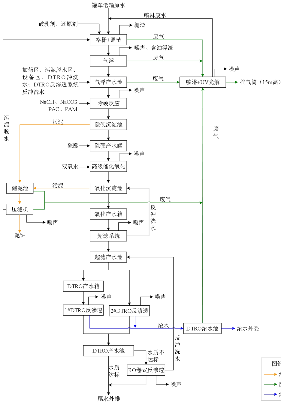
图 5-2 遂宁市博通科技有限公司工业废水处理厂一期工程废水处理流程图
