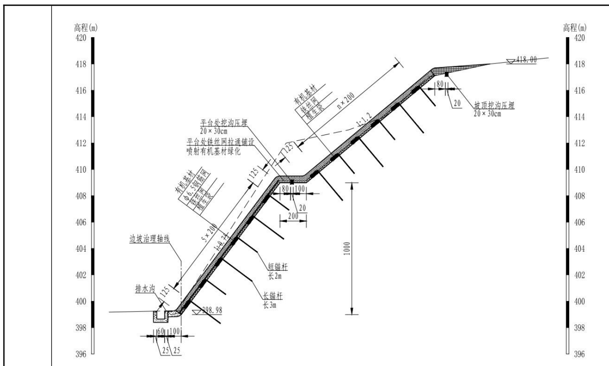
图 2-2 挂双网喷射有机基材绿化典型设计图
