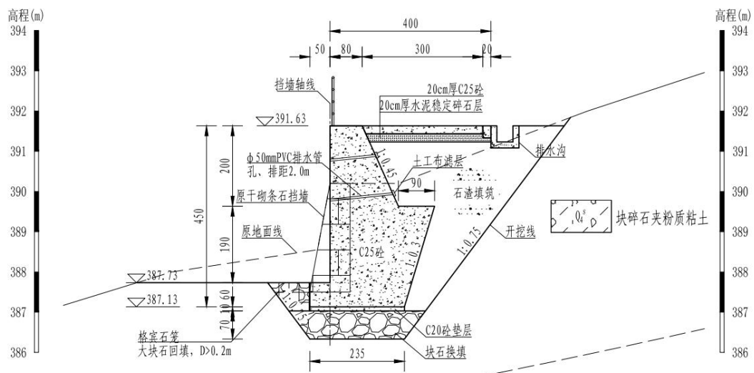
图 2-1 衡重式挡墙典型设计图
