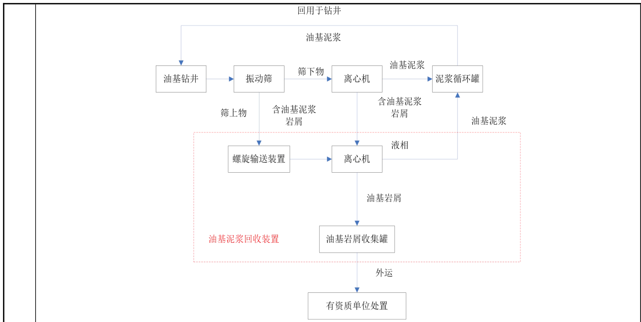
图 2.8-9 油基泥浆处理流程示意图
