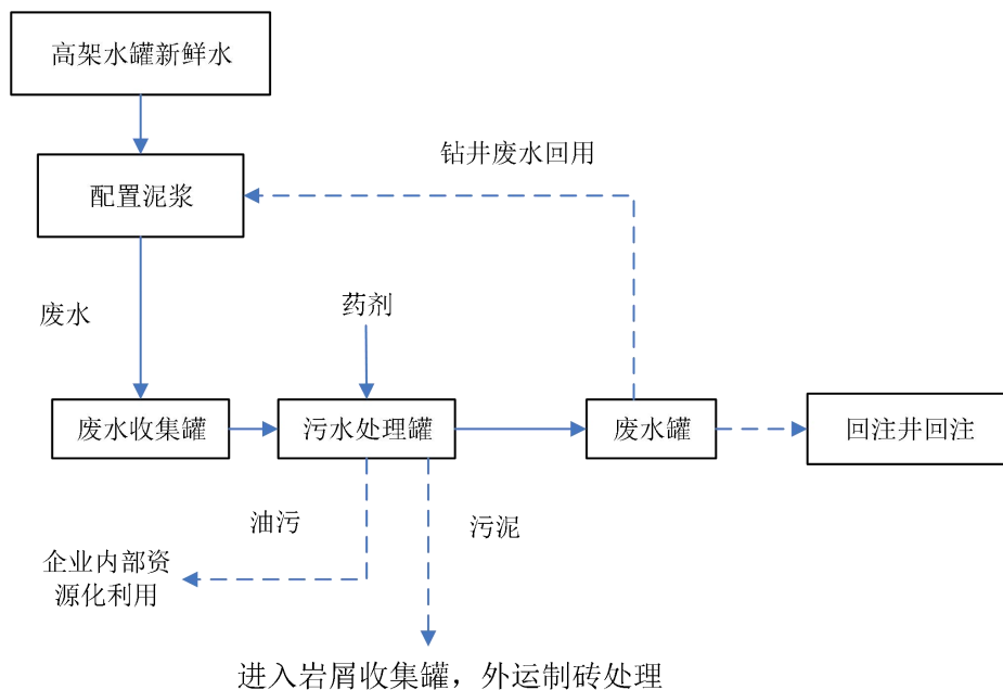
图 5.1-1 钻井作业废水预处理流程示意图
