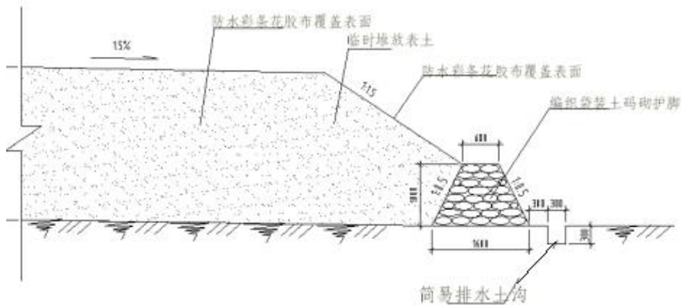
图 2.6-1 表土临时堆放场示意图
